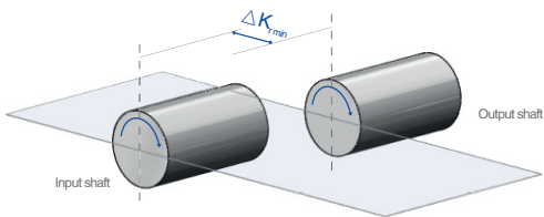
Figure1. 为确保施密特联轴器运转所需最小偏心量，输出轴处于水平方向Offset。
