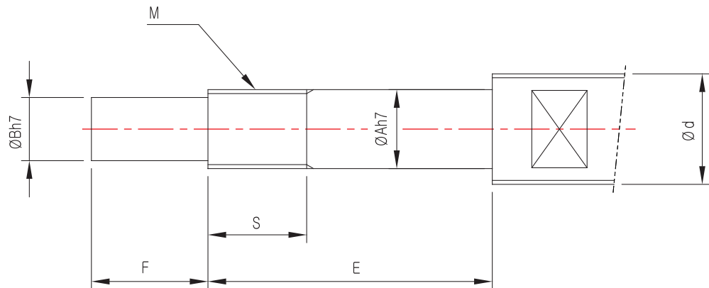
滚珠螺杆固定端轴端推荐形状
