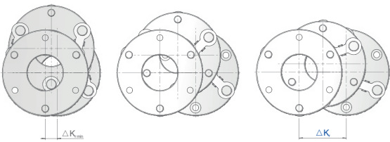
Figure4. 两轴间偏心(Radial offset)最小与最大时的中间Disk位置变化
