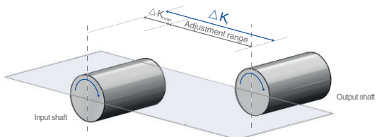
Figure3. 最大径向容许位移(Maximum Radial Offset \Delta K_r )。
